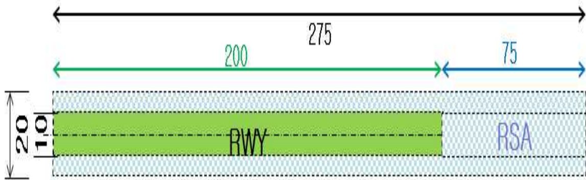
[그림 20] 활주로 시단 한쪽에 안전구역을 설치한 활주로 평면도
