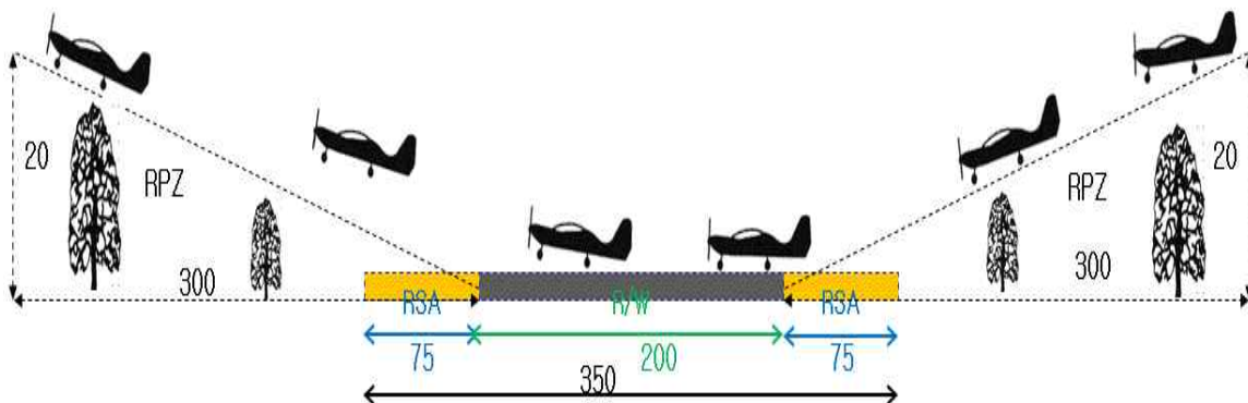
[그림 16] 활주로 양쪽에 안전구역을 설치한 활주로에서의 이착륙 형상
